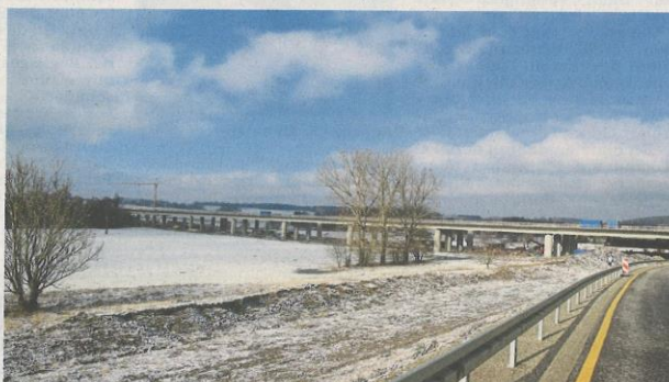
Massiv spannt sich die knapp 600 Meter lange Brücke über das Isental. Im Herbst 2019 soll hier der Verkehr zwischen München und Passau fließen.
